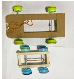
ゴム動力自動車
